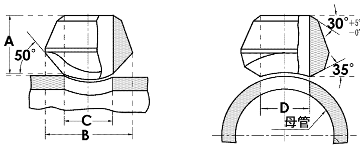
同径ウエルドオーレット
